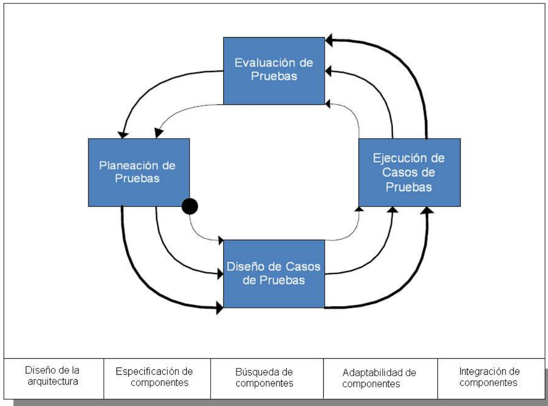
FASES DEL DESARROLLO DE SOFTWARE BASADO EN COMP. Fases del Procedimiento
